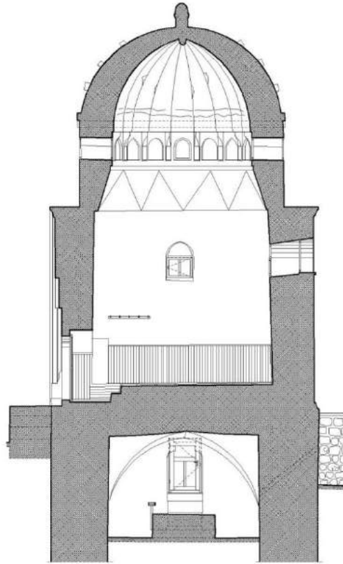
Şekil 5. Hasbey Dar'ül Huffazı'nın D-D kesiti
