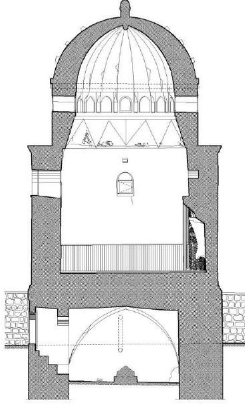
Şekil 4. Hasbey Dar'ül Huffazı'nın A-A kesiti
